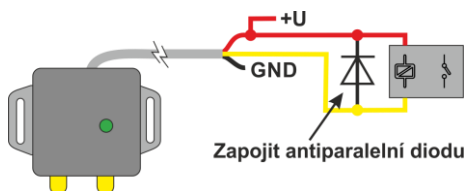
Zapojení s relé – galvanické oddělení, platí pro Výstup 1 (NC) i Výstup 2 (NO)
